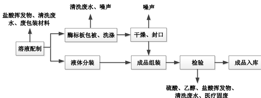
图 2-2 酶联免疫法产品生产工艺流程及产污环节图
